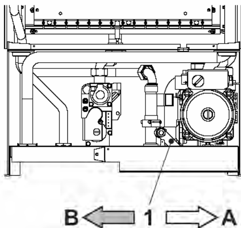
рис. 4 - Кран для заливки воды
