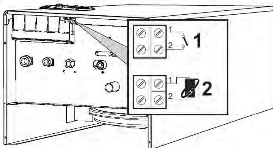
рис. 6 - Доступ к клеммной коробке
