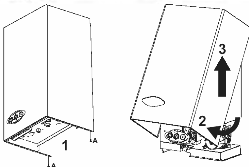
рис. 16 - Снятие кожуха
