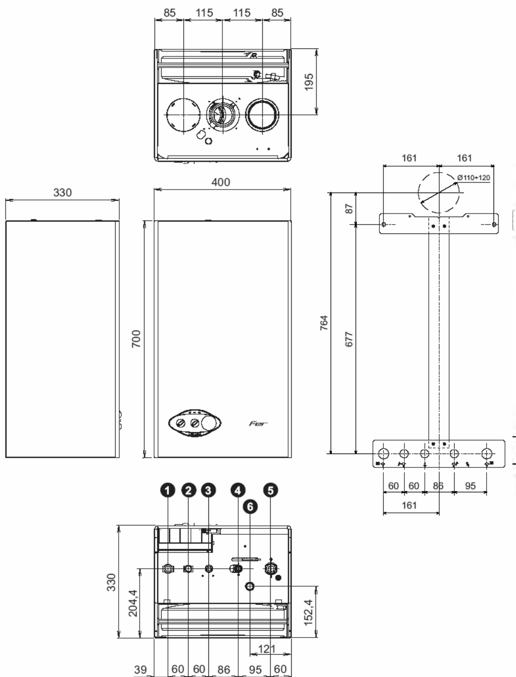
рис. 18 - Габаритные размеры и подключения
