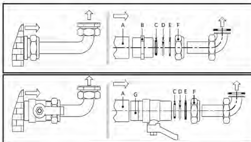
рис. 5 - Соединительный комплект
