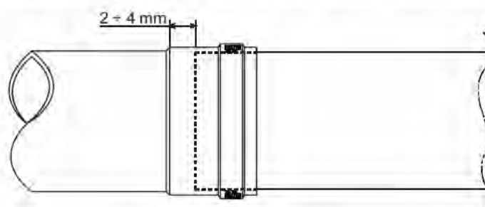
рис. 7 - Тепловое расширение
