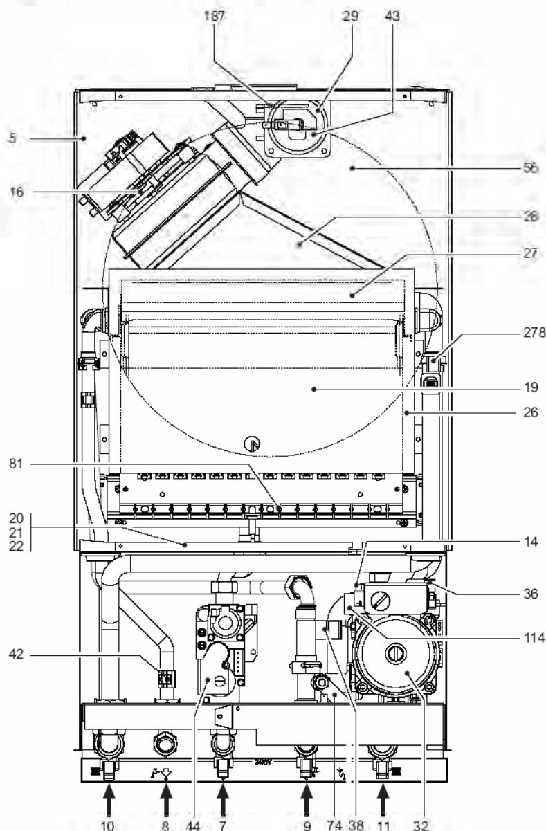
рис. 19 - Общий вид
